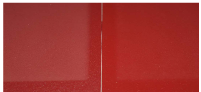
Retención de brillo: envejecimiento acelerado QUVB 600h - Alesta® AP izquierda/Alesta® SD derecha
